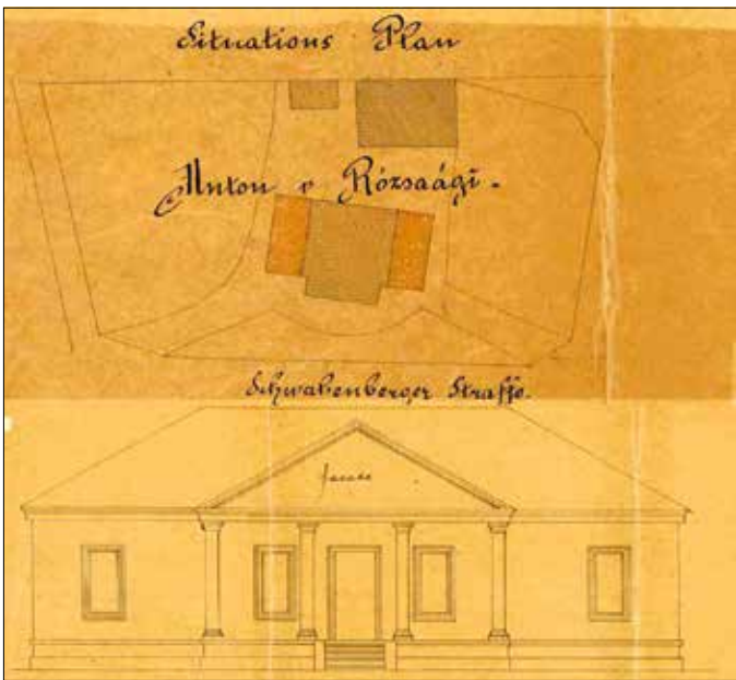
Rózsáagi Antal 1873-as bővítési tervei
